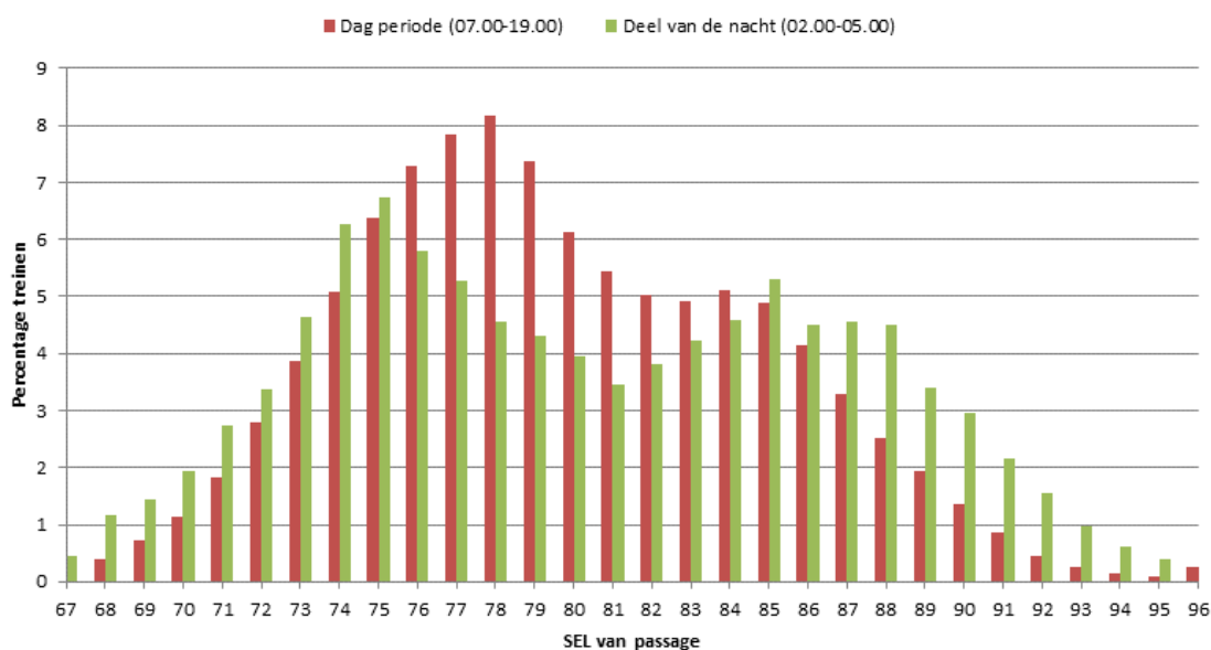
Figuur 15: spreiding in SEL-geluidsniveau van treinpassages. De groene balken zijn representatief voor de spreiding in goederentreinen.
