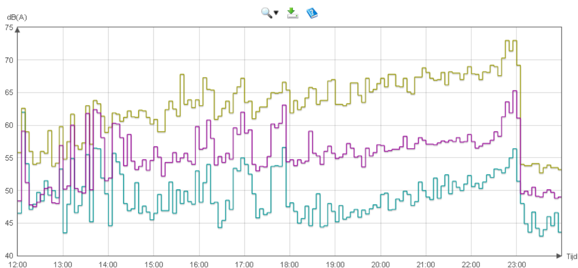
Figuur 26: overzicht gemeten geluidsniveaus rond van Lakedance voor locatie zuidoost (beige) en villawijk (paars) en Batadorp (licht blauw). De locatie langs het spoor heeft een vrijwel identiek geluidniveau als bij Villawijk.
