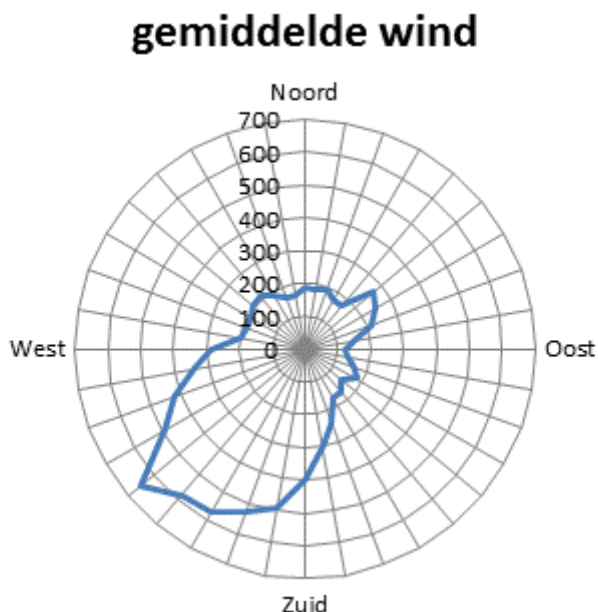
Figuur 32: overzicht aantal uren gedurende de dagperiode en over de meetperiode dat een bepaalde windrichting voorkwam. Er is gekeken in stappen van 10 graden (36 windrichtingen).
